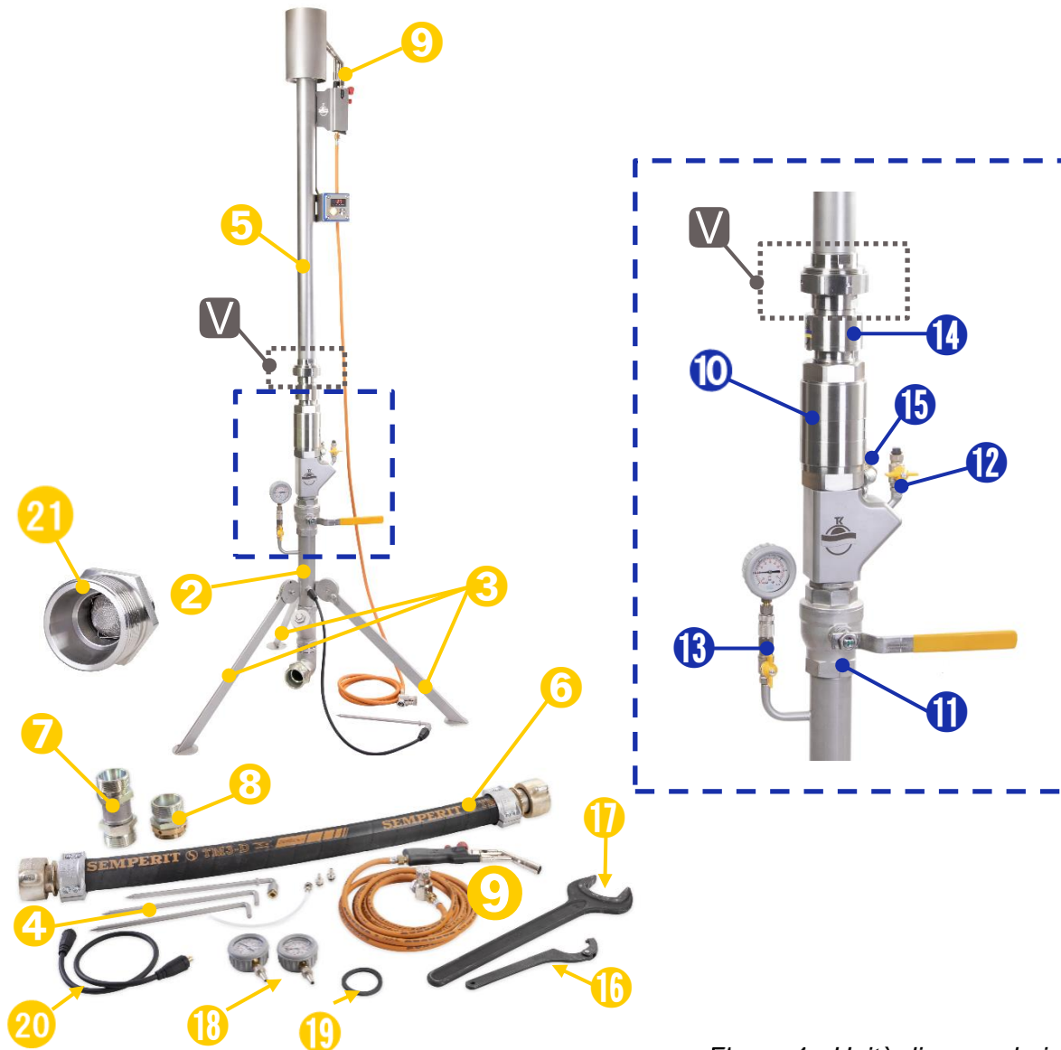
Figura 3: Componenti di sistema
