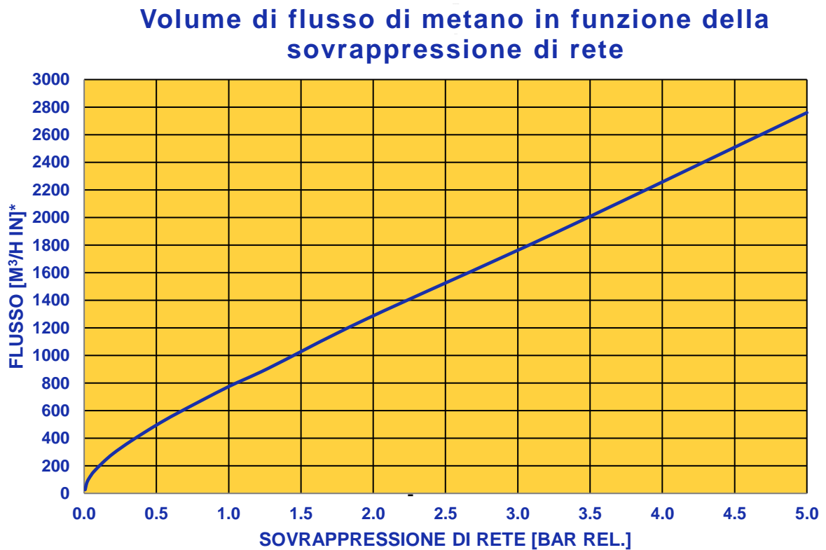
Figura 5: Volume di flusso di metano in funzione della sovrappressione di rete
