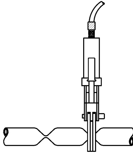
Bild 4: Zweite Quetschung
