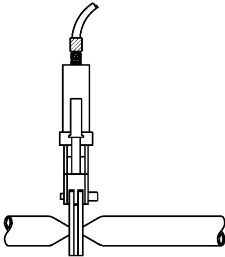
Bild 3: Erste Quetschung
